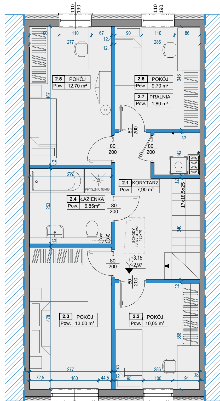
PIĘTRO
